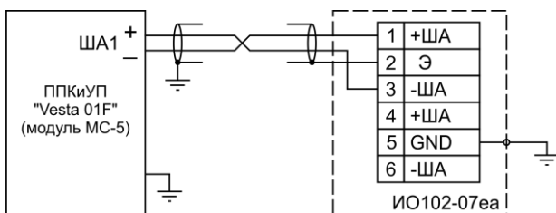
Рисунок 6 - Общая схема подключения извещателей ИО102-07ea в двухпроводную АЛС “ША” ППКиУП “Vesta 01F” или модуля “МС-5”.
