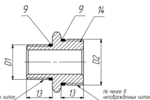
б) Переход взрывозащищенный КВВ-П-Н
