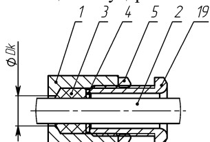
д) открытая прокладка кабеля в кабельном вводе КВВ
