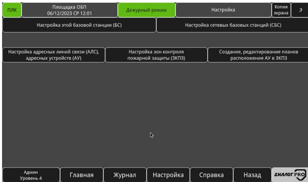
Рисунок 3.50 – Окно «Настройки»
