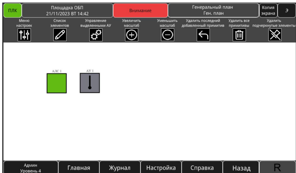
Рисунок 3.93 – элементы-АУ
