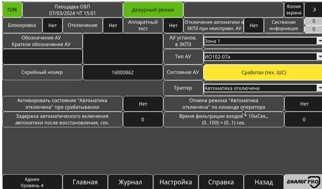
Рисунок 3.86 – Конфигурация «ИО102-07а-ДПРО»
