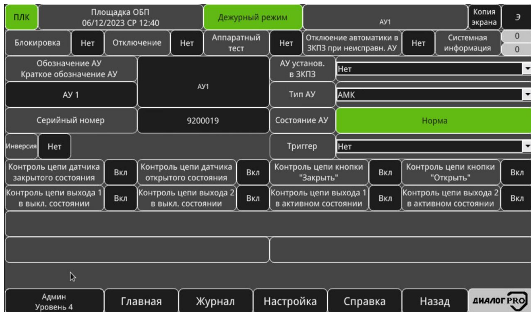
Рисунок 3.77 – Конфигурация «АМК»
