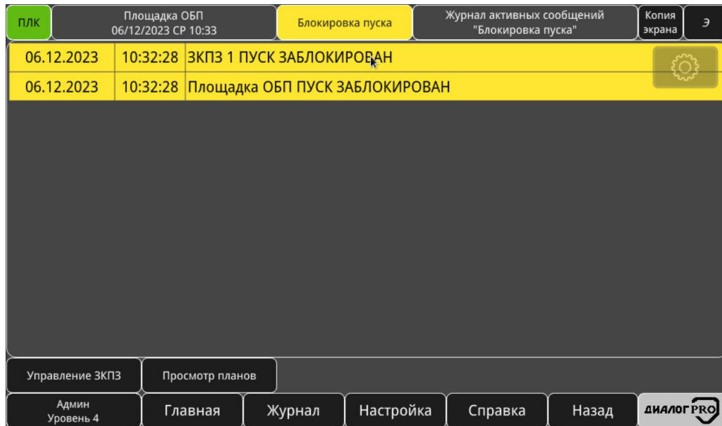
Рисунок 3.31 – Окно «Журнал активных сообщений «Блокировка пуска»
