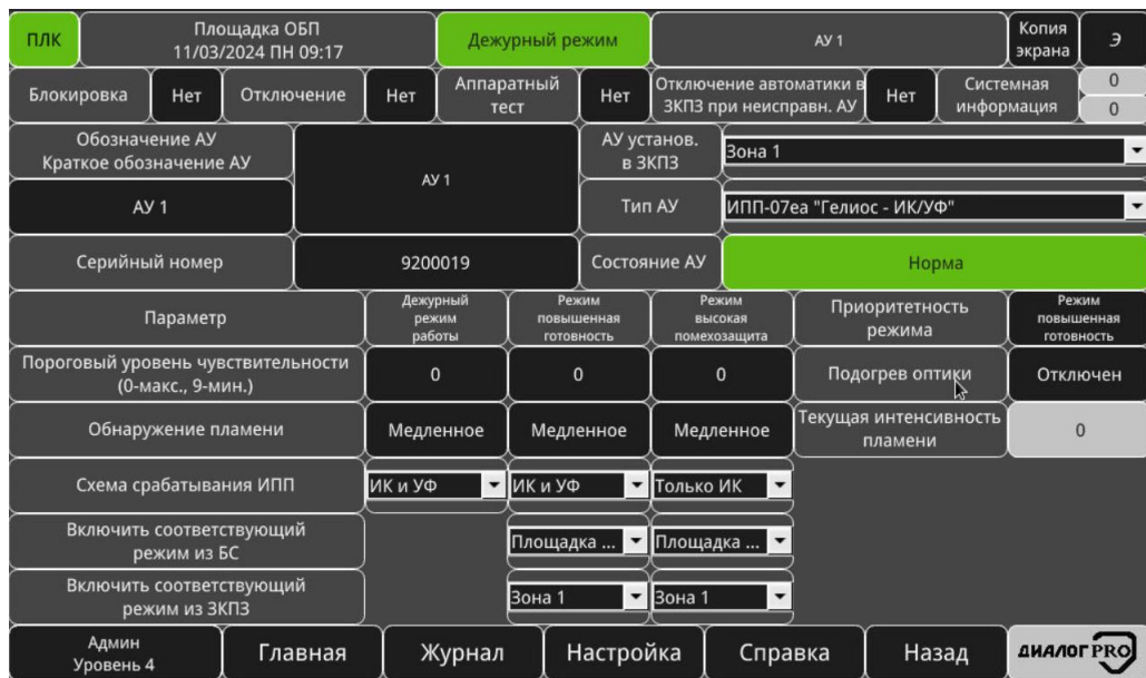
Рисунок 3.74 – Конфигурация «ИПП-07еа «Гелиос-3 ИК/УФ» Д1-ДПРО»
