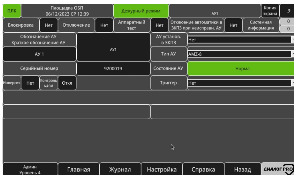
Рисунок 3.66 – Конфигурация АМZ-8, АМС-42/44 вход, АМ вход
