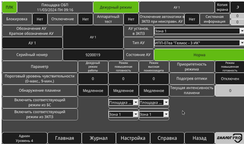
Рисунок 3.73 – Конфигурация «ИПП-07еа «Гелиос-3 ИК» Д1-ДПРО»
