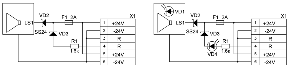
а) BC-07e-Eх-3-24VDC
