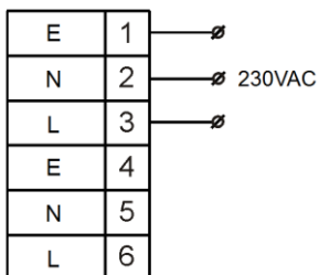
Рисунок 3. Схемы подключения оповещателей BC-07e-Eх-24VDC.
