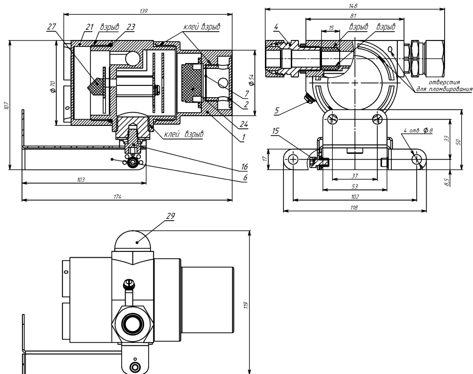
а) Габаритные размеры оповещателя WS-07e-Ex-3(И).
