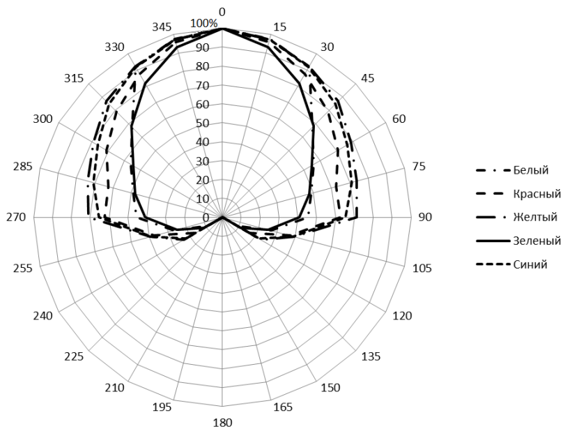
Рисунок В.1 Диаграммы направленности звукового сигнала оповещателя
