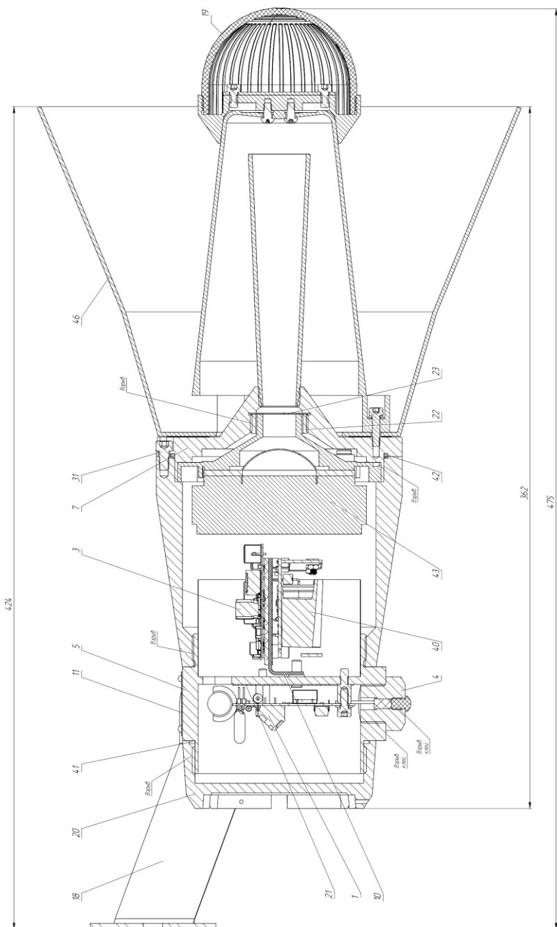
б) Габаритный чертеж оповещателя ВС-07е-3М/СД
