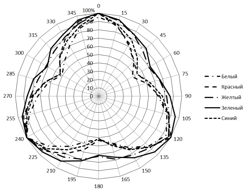
Рисунок В.2 – Нормированная диаграмма силы света ВС-07с-3М в зависимости от цвета колбы оповещателя
