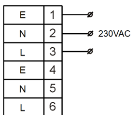
Рисунок 3. Схемы подключения оповещателей BC-07e-O-24VDC.
