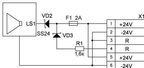
а) BC-07е-О-3-24VDC
