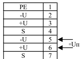
в) BC-07е-СЛ-24VDC
