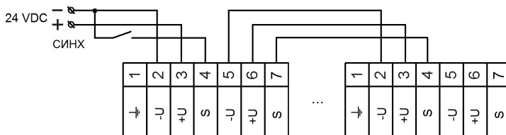
Рисунок 6. Использование режима синхронизации в оповещателе BC-07е-О-СЛ-24VDC.
