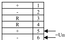
а) BC-07е-3(И)-24VDC
