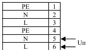
а) BC-07е-230VAC
