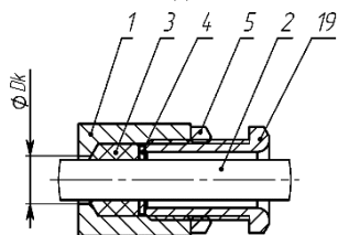
д) открытая прокладка кабеля в кабельном вводе KBВ
