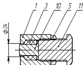
ж) монтаж заглушки KBГ
