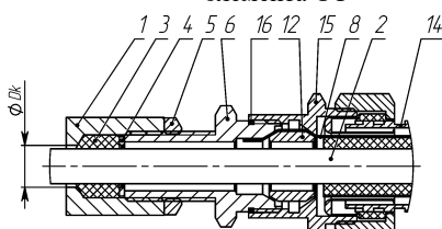
и) монтаж бронированным кабелем в металлорукаве в кабельном вводе КВЕМ
