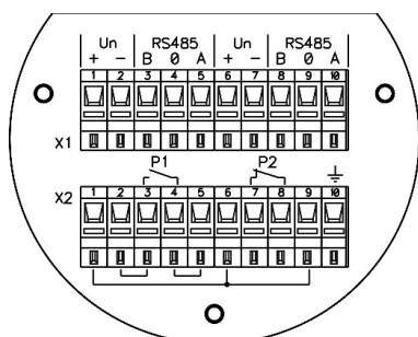
а) Плата клемм извещателя ИППИ-07ea-RS
