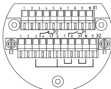
б) Плата клемм извещателя ИППИ-07ea-RS-4/20мА
