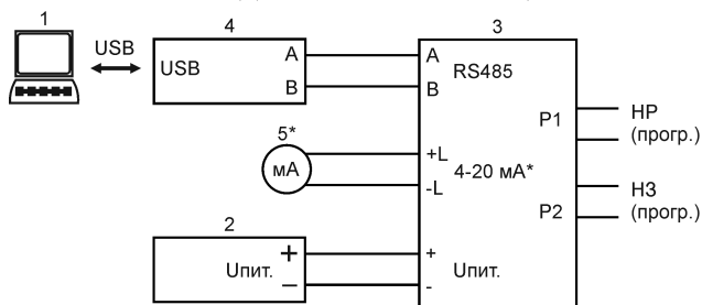
Рисунок Б.1 Функциональная схема подключения извещателя ИППИ-07ea-RS к ПК для конфигурирования или проверки работоспособности
