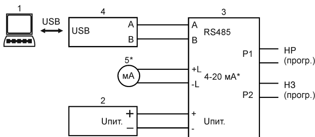
Рисунок Б.1 Функциональная схема подключения извещателя ИПП-07ea-RS к ПК для конфигурирования или проверки работоспособности
