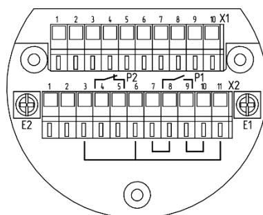
б) Плата клемм извещателя ИПП-07еа-RS-4/20мА
