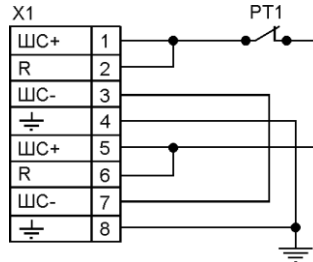
Рисунок В.1 - Схема электрическая извещателя ИП103-2/1-ТР
