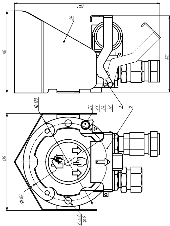
б) Внешний вид извещателя ИП535-07е-В-О
