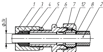
в) монтаж бронированным кабелем в кабельном вводе КББ17
