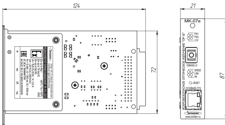
Рисунок 1. Габаритные размеры медиаконвертера МК-07е-22ЕХХ.
