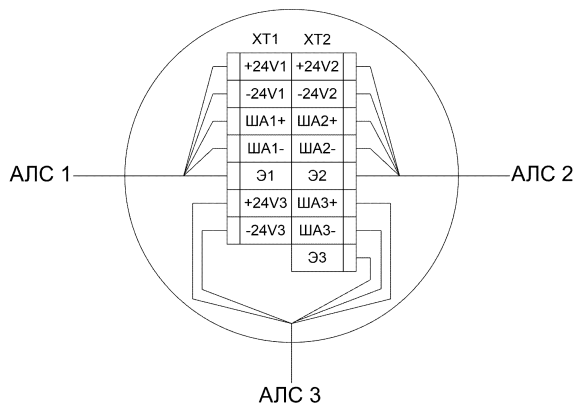
Рисунок 2 – Схема внешних подключений с отводом линий интерфейса и питания
