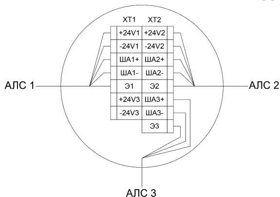
Рисунок 3 – Схема внешних подключений с отводом линии интерфейса
