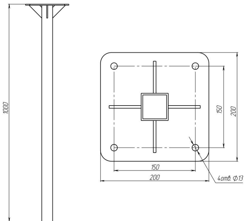
Рисунок 5 – Габаритные и присоединительные размеры закладной стойки СП-013
