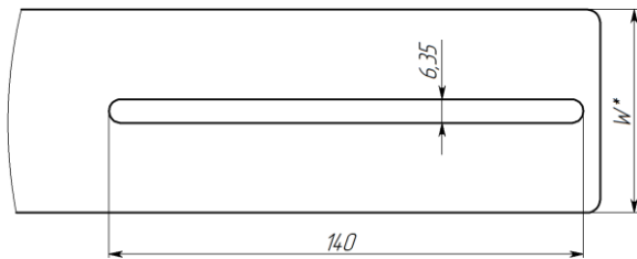
Рисунок А.7 - Направляющая с пазом для установки видеокамеры в термокожух ТВК-07-Н/С
