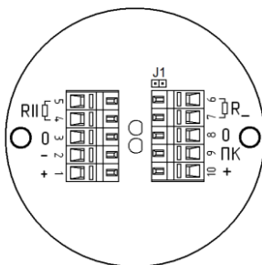
Рисунок 4 - Внешний вид платы УДП ИП535-07е-“ПУСК”-И2
