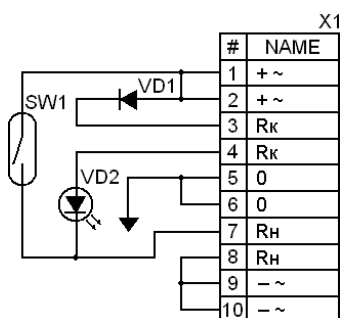
а) Электрическая схема устройства УДП ИП535-07е-“ПУСК”-И1
