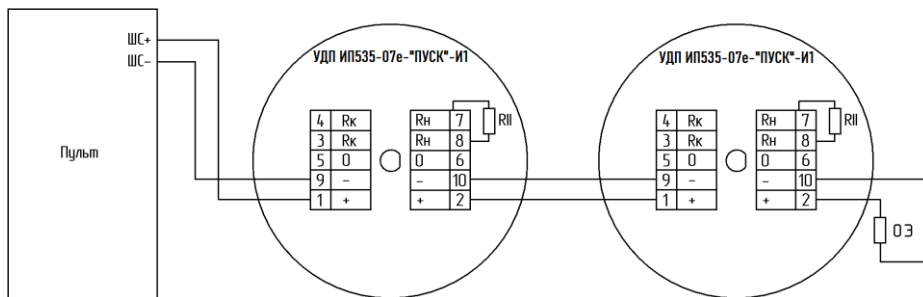
Рисунок 7 - Схема подключения УДП ИП535-07е-“ПУСК”-И1 в шлейф приборов
