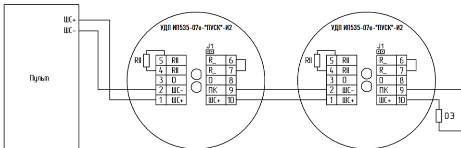
в) Схема подключения на замыкание
