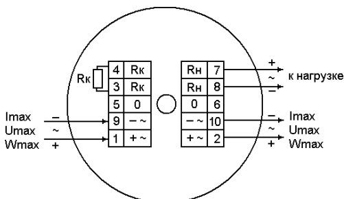
б) Условная схема подключения УДП ИП535-07е-“ПУСК”-И1 при работе непосредственно на нагрузку
