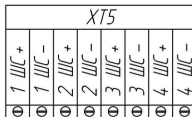
Контролируемые дискретные входы (ШС) схема подключения в таблице 1
