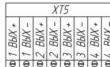
Контролируемые дискретные выходы (ШС) схема подключений в таблице 2 макс. коммутируемый ток не более 2 А на канал
