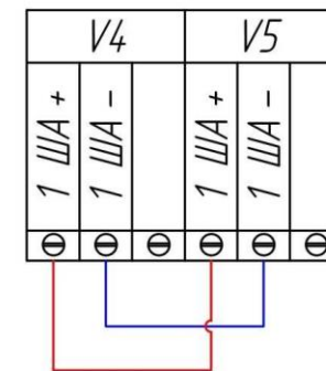
АЛС "ША" №1 (кольцо)
