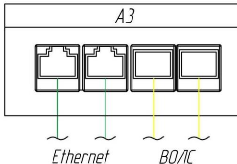
Резервированная кольцевая линия связи для объединения базовых станций в сеть
