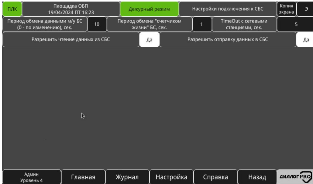
Рисунок 3.54 – Окно «Настройка подключения СБС»
