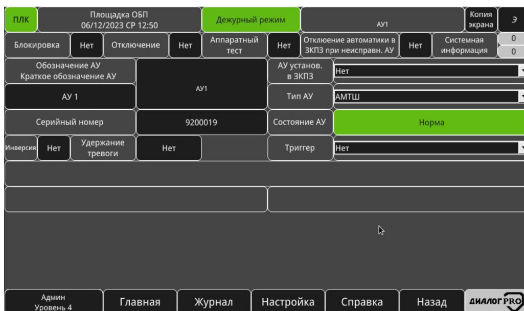
Рисунок 3.109 – Конфигурация «АМТ», АМД», «АМТШ», АМДШ»
