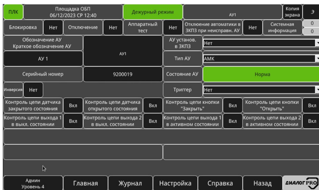
Рисунок 3.101 – Конфигурация «АМК»
