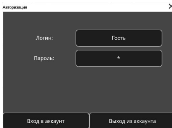
Рисунок 3.17 – Окно «Авторизация»
