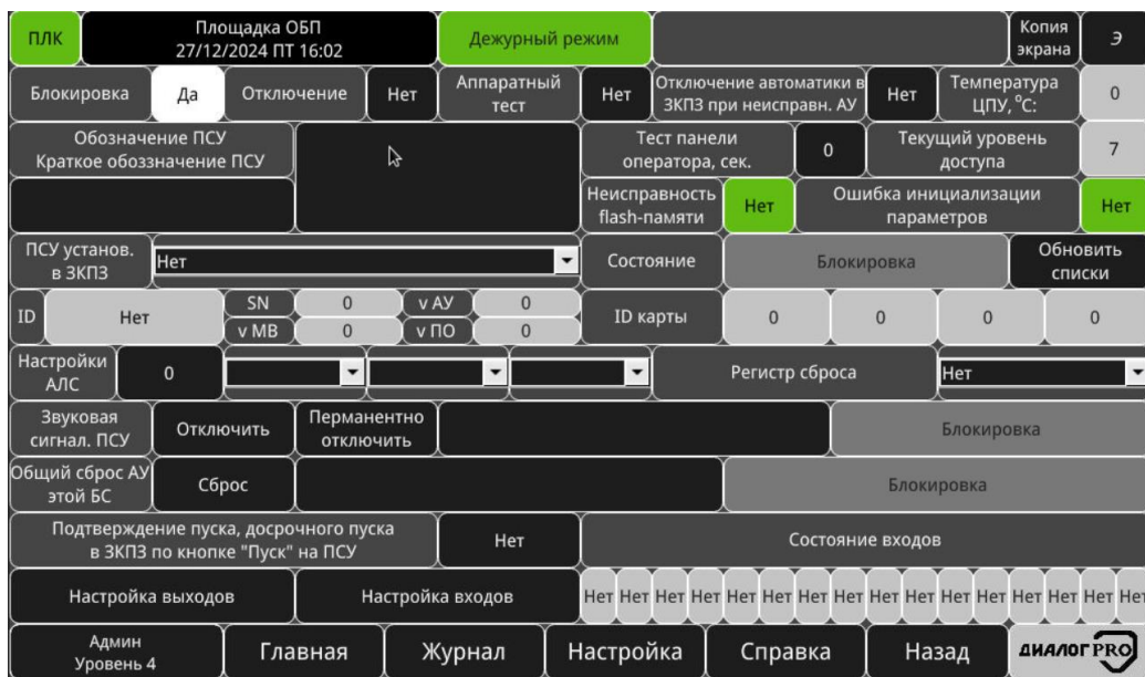
Рисунок 3.63 – Окно «Панель сигнализации и управления (ПСУ)»
