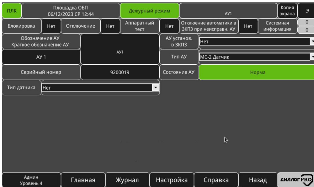
Рисунок 3.108 – Конфигурация «МС-2 Датчик»
