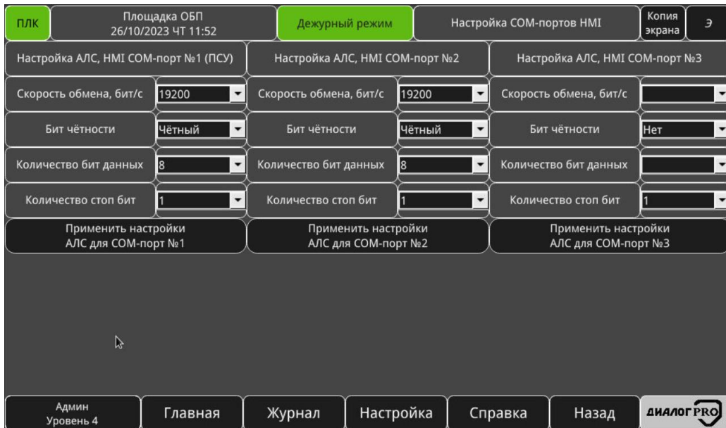
Рисунок 3.57 – Окно «Настройка СОМ-портов»
