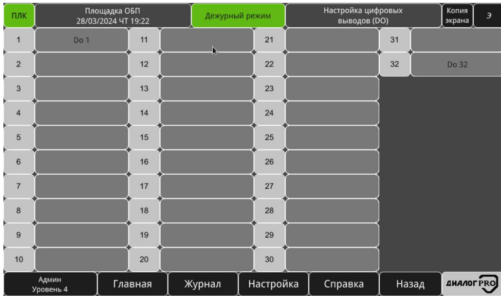
Рисунок 3.75 – Окно «Настройка цифровых выводов (DO)»
