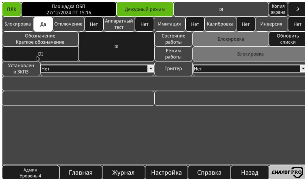
Рисунок 3.78 – Окно конфигурирования цифрового ввода
