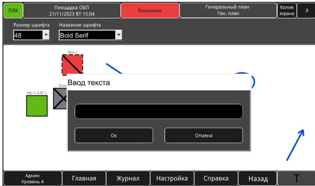
Рисунок 3.128 – панель параметров текста и всплывающее окно для ввода текста
