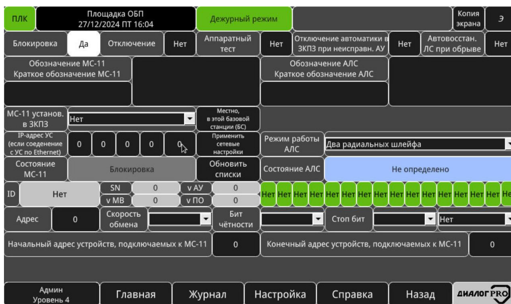
Рисунок 3.72 – Окно «Контроль АЛС RS-485 до компонентов БС (МС-11)»
