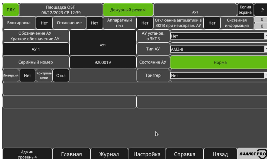
Рисунок 3.99 – Конфигурация АМЗ-8, АМС-42/44 вход, АМ вход
