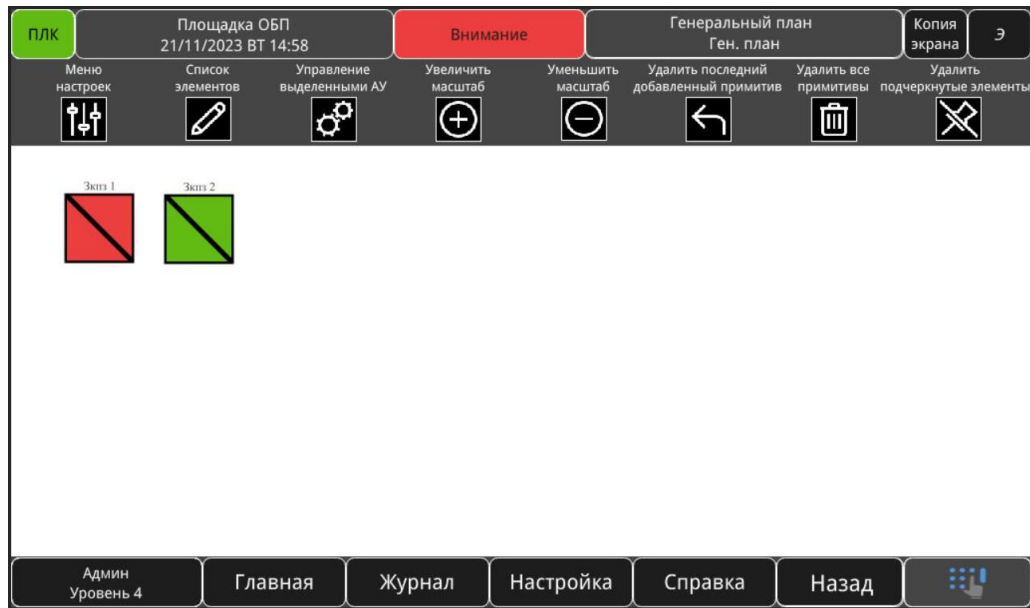
Рисунок 3.120 – элементы-ЗКПЗ
