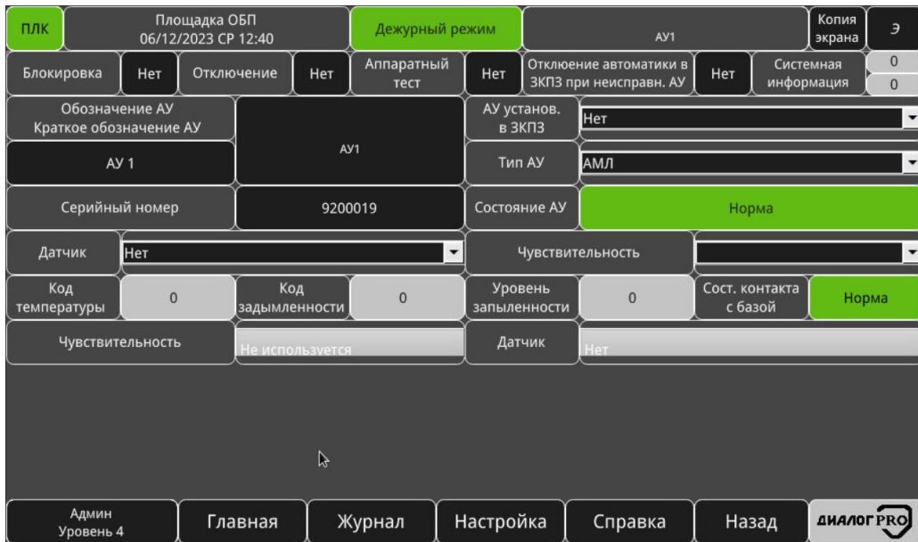
Рисунок 3.102 – Конфигурация «АМЛ»
