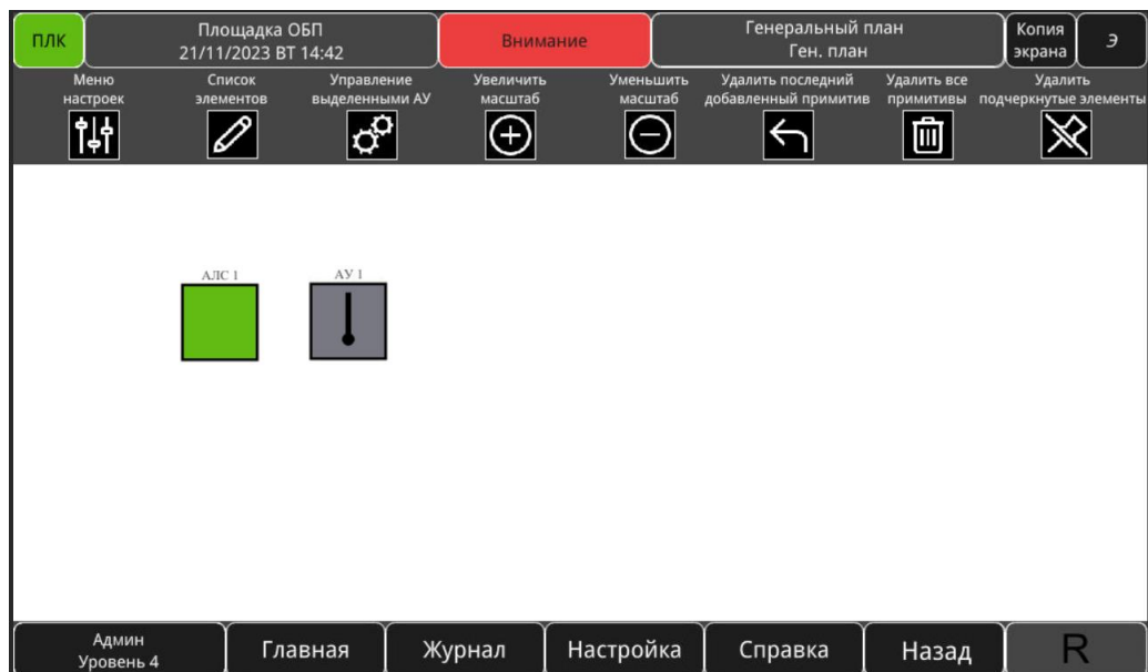
Рисунок 3.118 – элементы-АУ
