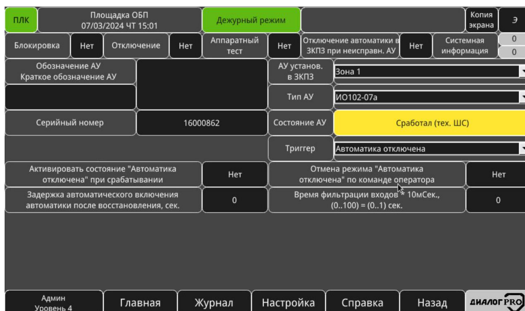
Рисунок 3.110 – Конфигурация «ИО102-07а-ДПРО»
