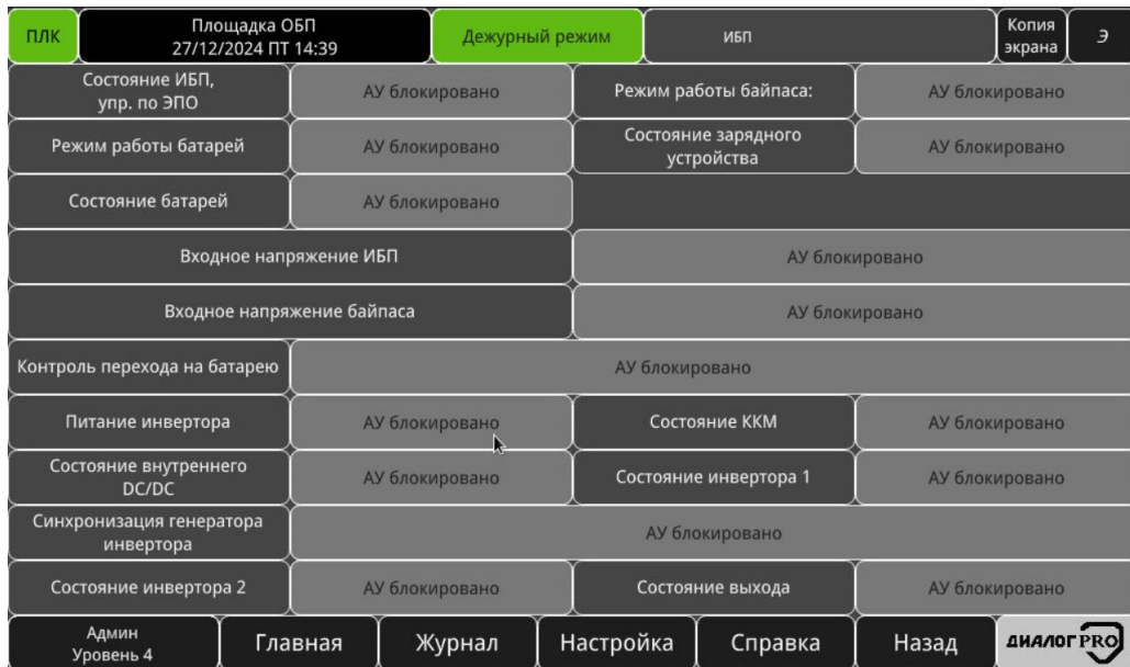
Рисунок 3.69 – Окно «Состояние»
