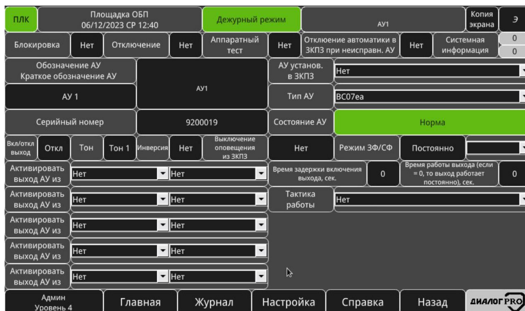
Рисунок 3.103 – Конфигурация «BC-07e-a-DPRO»
