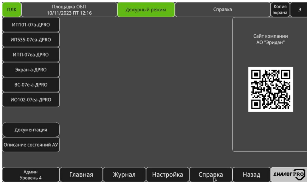
Рисунок 3.141 – Окно «Справка»
