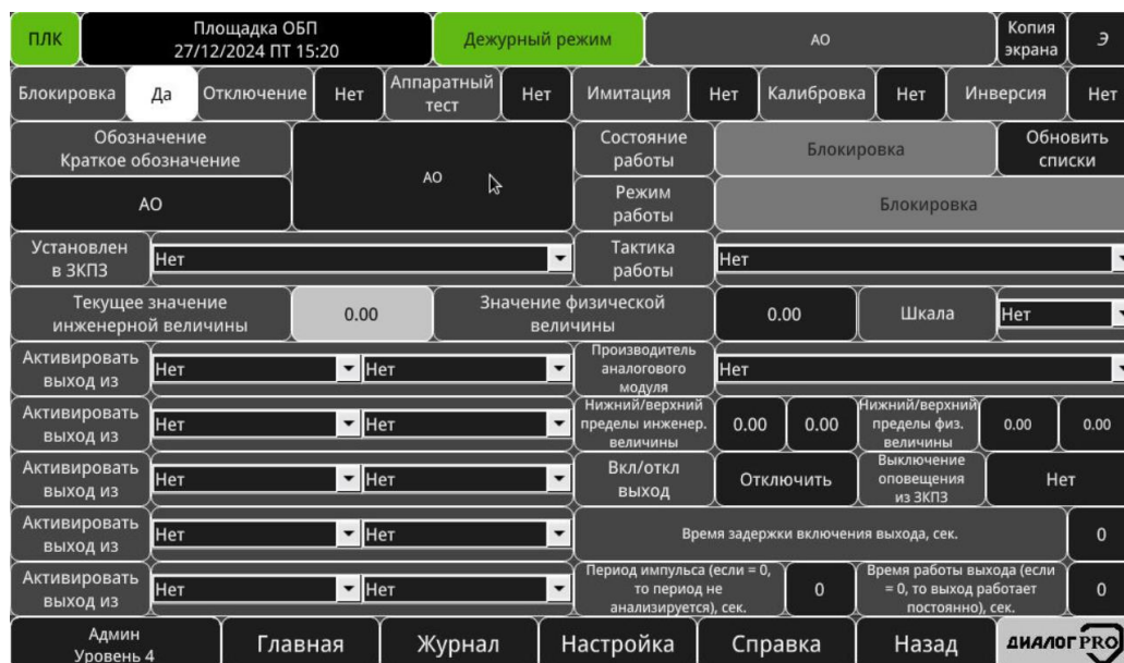
Рисунок 3.81 – Окно конфигурирования аналогового вывода
