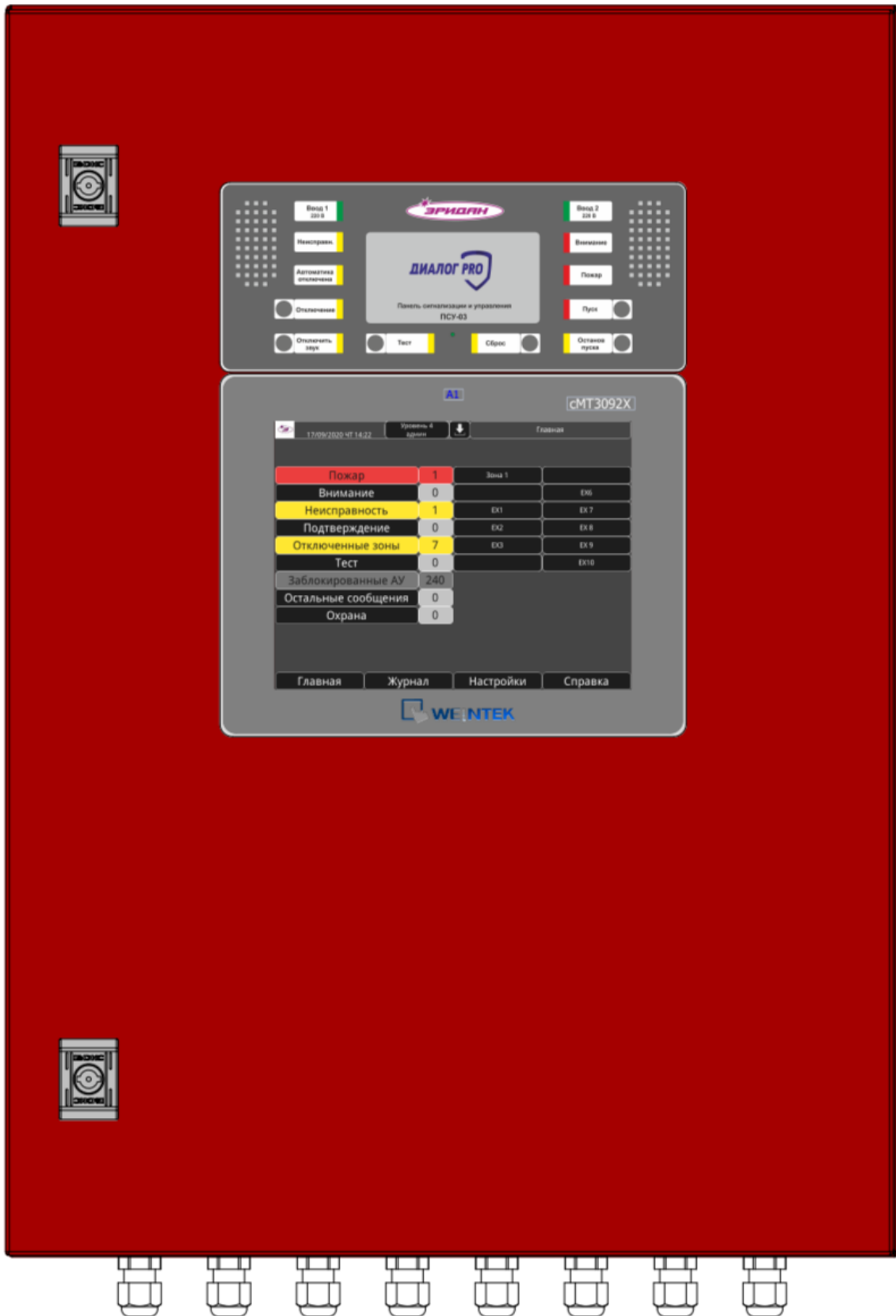
Рисунок Б.1 – Общий вид БС, исп. 1
