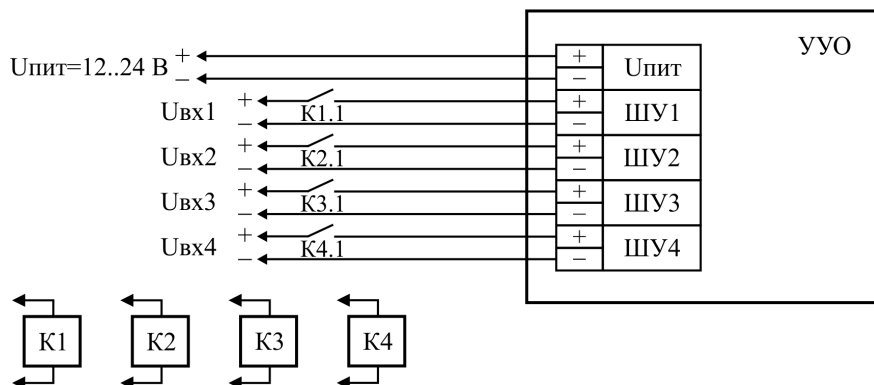
Рисунок 11. Пример схемы подачи внешних управляющих сигналов на УЮ-RGB через транзисторные ключи.
