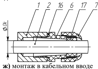
ж) монтаж в кабельном вводе КВП12 (для ЭКРАН-ИНФО-RGB-O)
