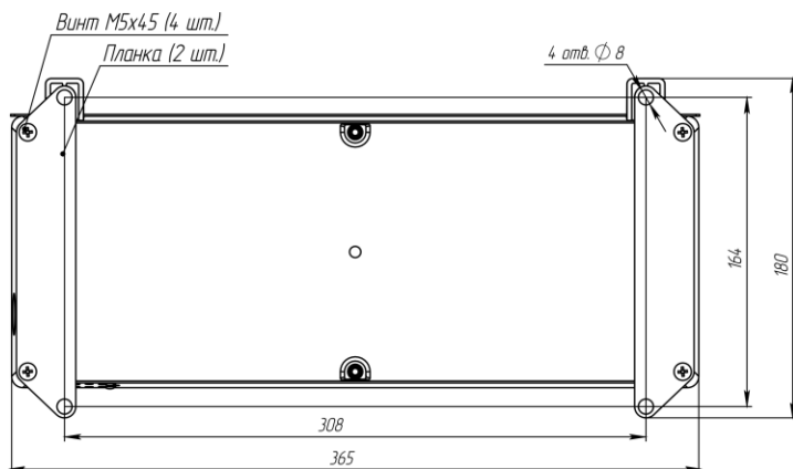
б) Монтаж планок АК-4Э (вид сзади)
