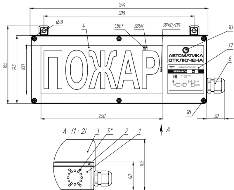
а) Внешний вид оповещателя
