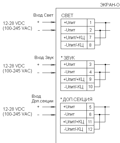
Рисунок 3. Схема подключения оповещателя ЭКРАН-О.
