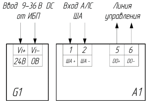
Рисунок 1 – Схема подключения УС
