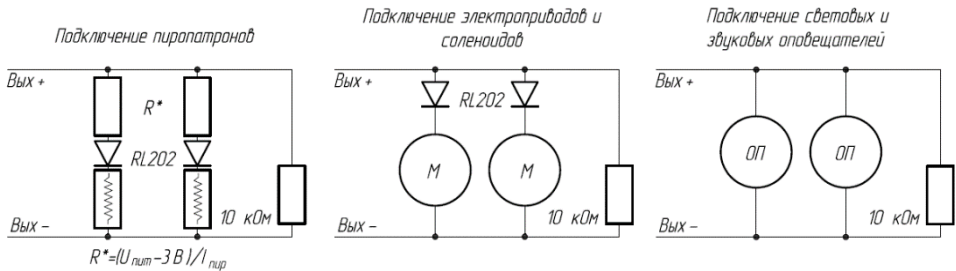
Рисунок 2 – Схема подключения линии управления
