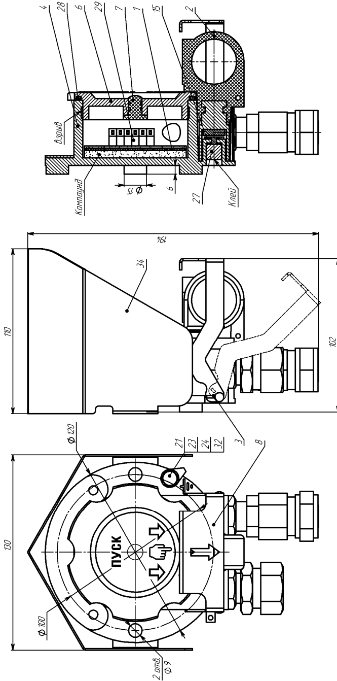
Рисунок 1. Внешний вид устройства пуска ИП535-07е-“ПУСК”.
