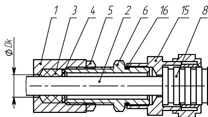
г) монтаж кабелем в металлорукаве KBМ
