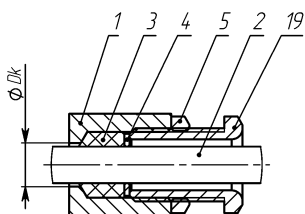
е) открытая прокладка кабеля в кабельном вводе КБО
