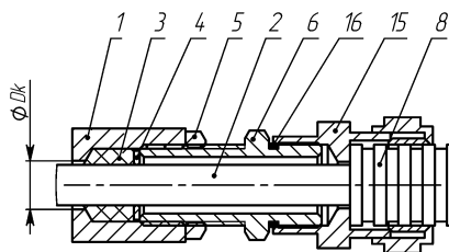
г) монтаж кабелем в металлорукаве КБМ
