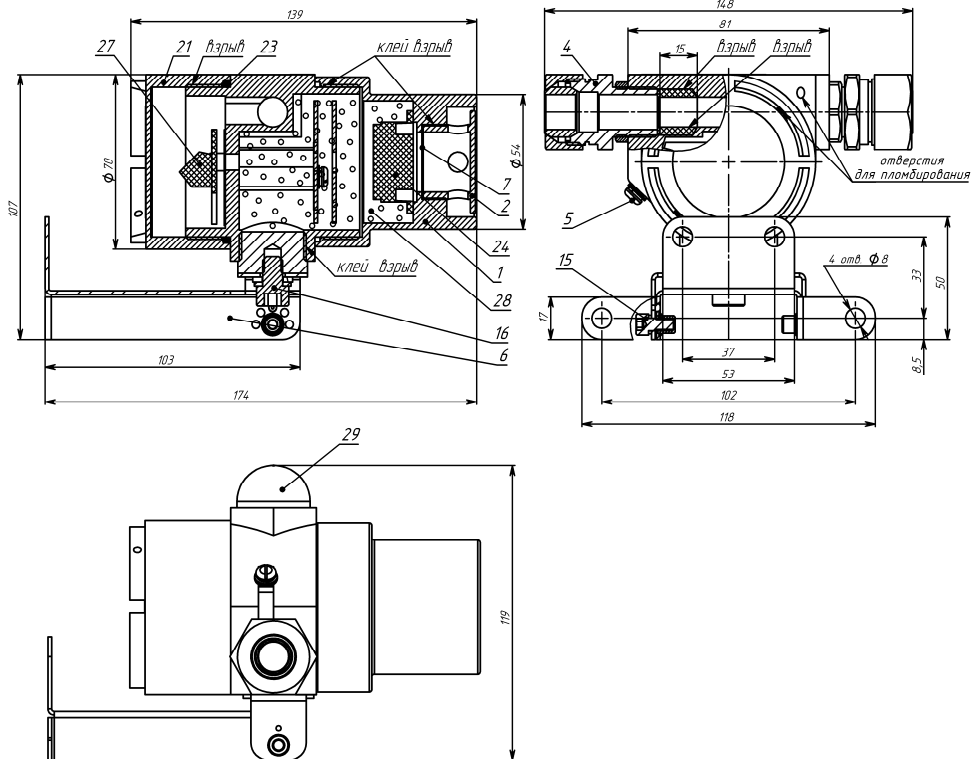
а) Габаритные размеры оповещателя WS-07e-Eh-3(И).
