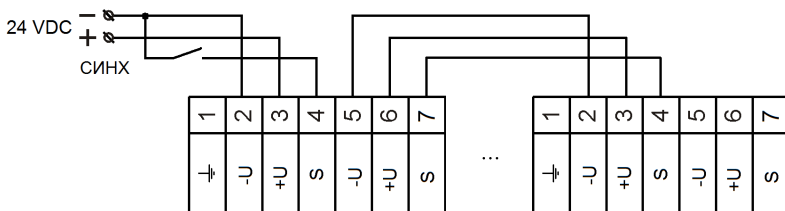
Рисунок 6. Выбор режима работы оповещателя BC-07e-Ex-3(I) с помощью переключателей J1 и J2.
